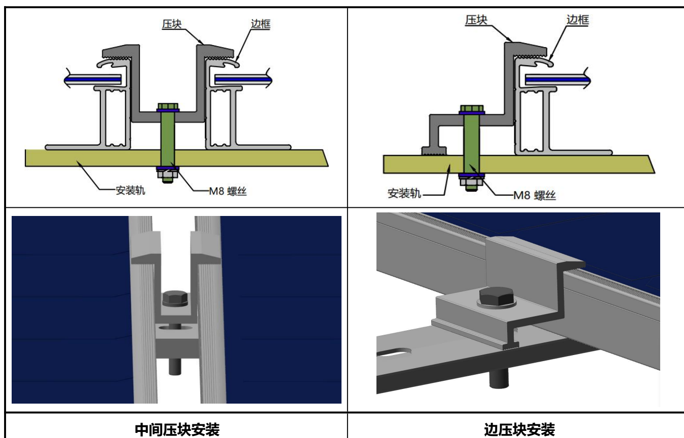
图2 压块安装示意图
