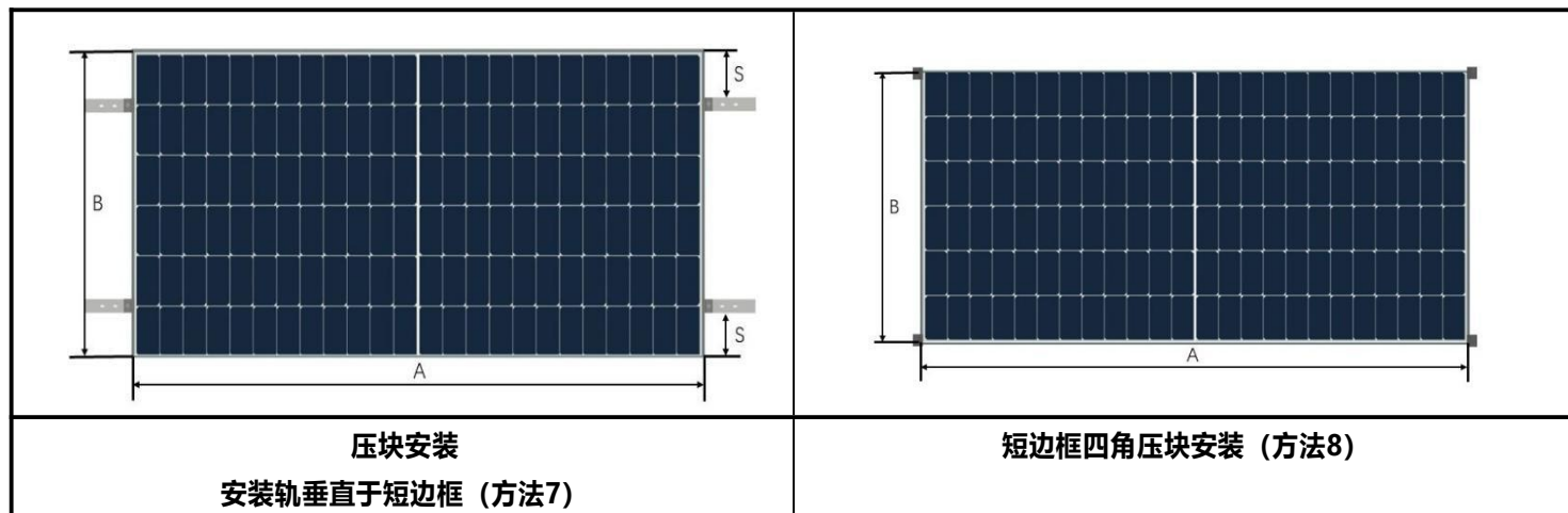
图4 双玻组件安装方式示意图
